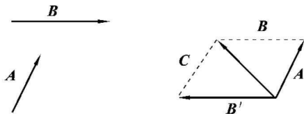
图 0-7 矢量的减法
