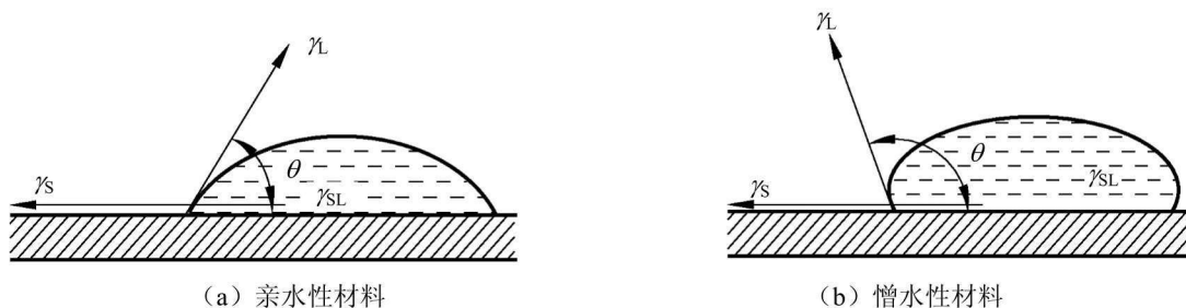
图 1.4 材料的湿润角示意图
