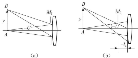
图 1-5 孔径光阑位置
