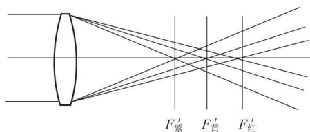
图 1-7 单透镜对无限远轴上物点白光成像
