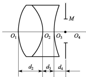
图 1-1 光学系统图
