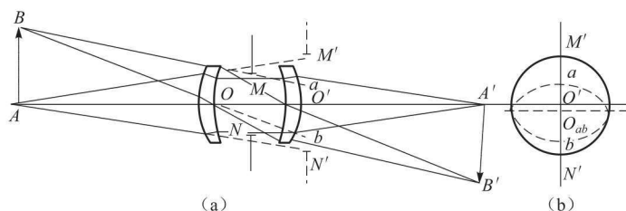
图 1-6 光学系统的渐晕
