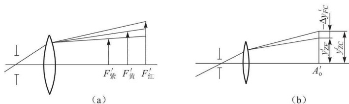
图 1-8 单透镜对无限远轴外物点白光成像
