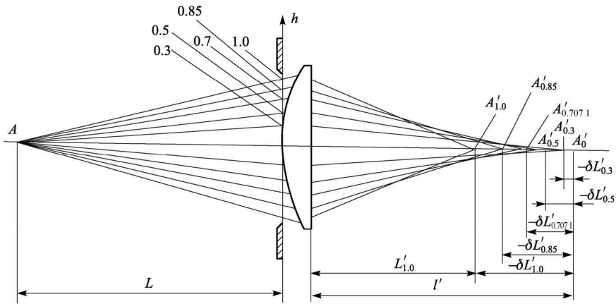
图 1-9 球差示意图
