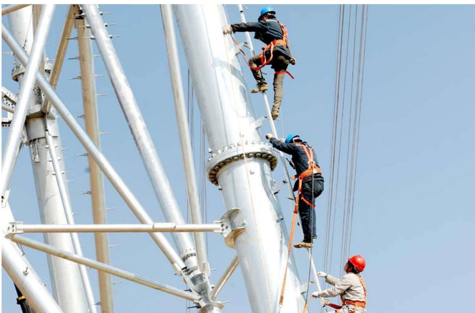
↘ 特高压电网工程作业现场
