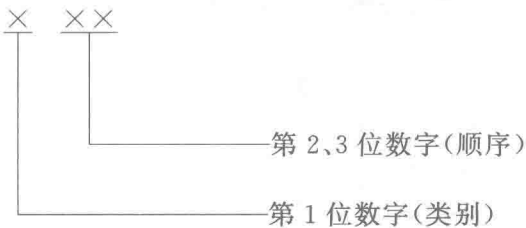
图 1 代码结构图
