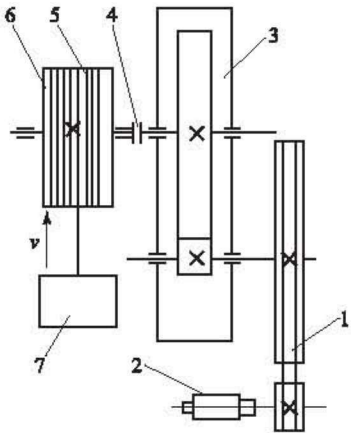
图 1-2 传动方案图
