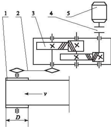
图 1—4 传动方案图
