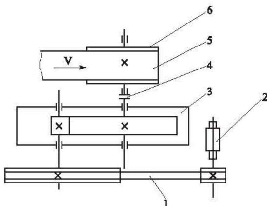
图 1-1 传动方案图
