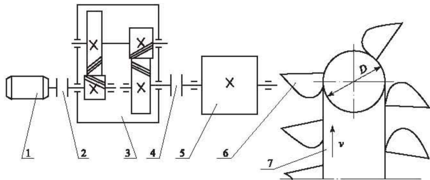
图 1.3 传动方案图
