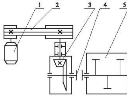
图 1-6 锥齿轮减速器传动方案图
