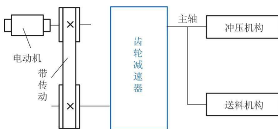
图 1-2 冲床的传动系统示意图
