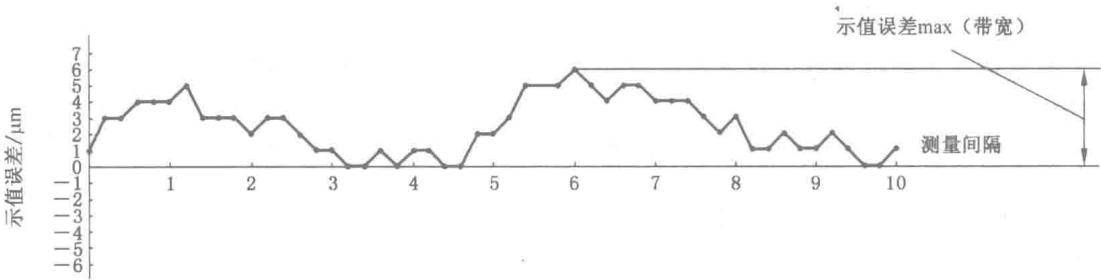
图 4 相对于浮动零位的示值误差(测量杆正行程曲线)示意图
