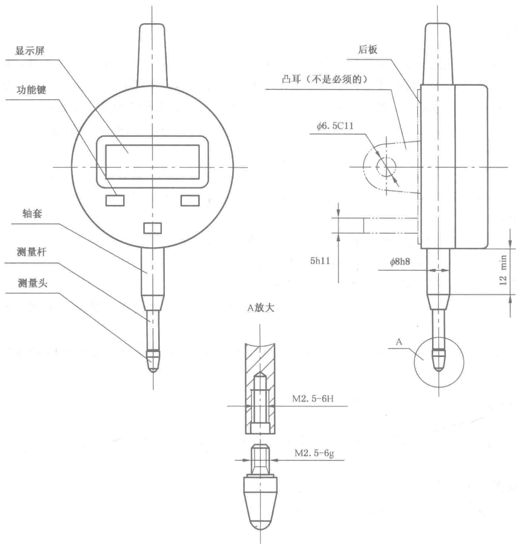
图 1 电子数显指示表的型式示意图
