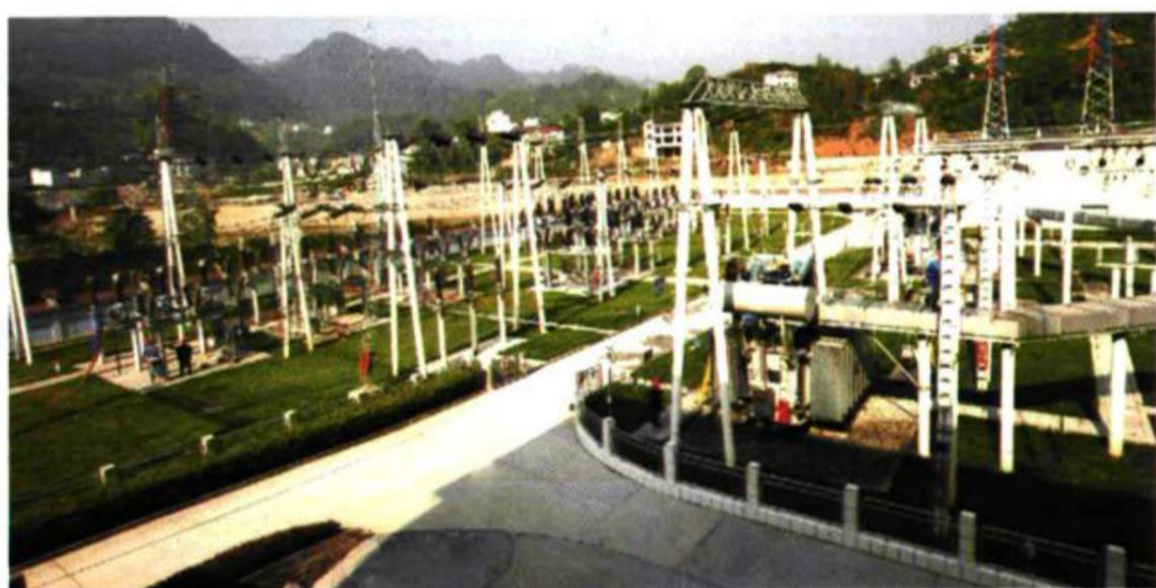
110千伏莲花坝变电站 (2009年摄)
