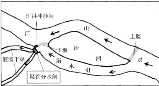
第 33 题图 姜席堰平面示意图
