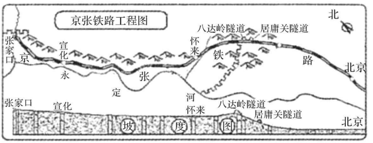
京张铁路工程图
