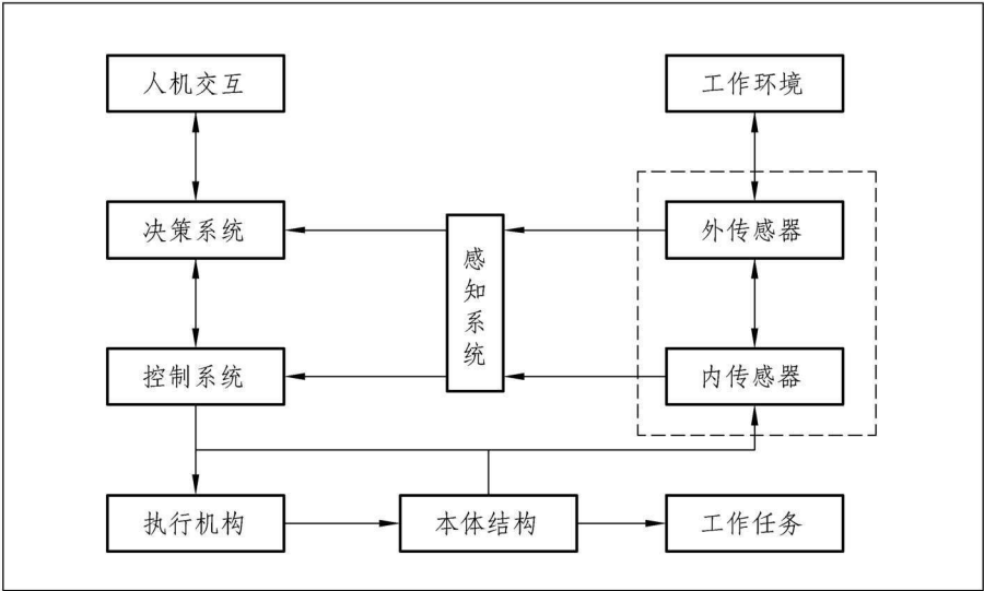
图 1-1 服务机器人的系统构成
