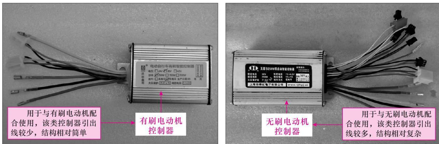
图 1-6 常见控制器的实物外形
