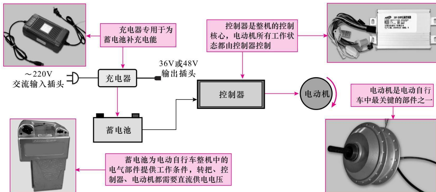
图 1-11 电动自行车四大件的关系示意图
