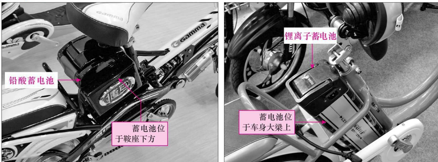
图 1-7 电动自行车中蓄电池的实物外形
