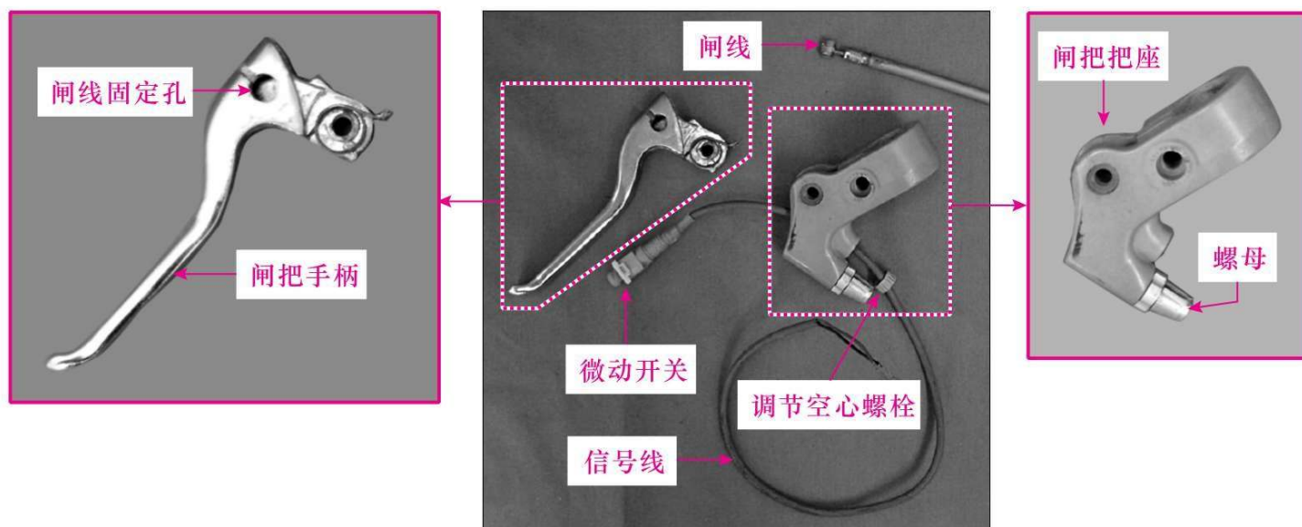
图 1-15 闸把的结构组成
