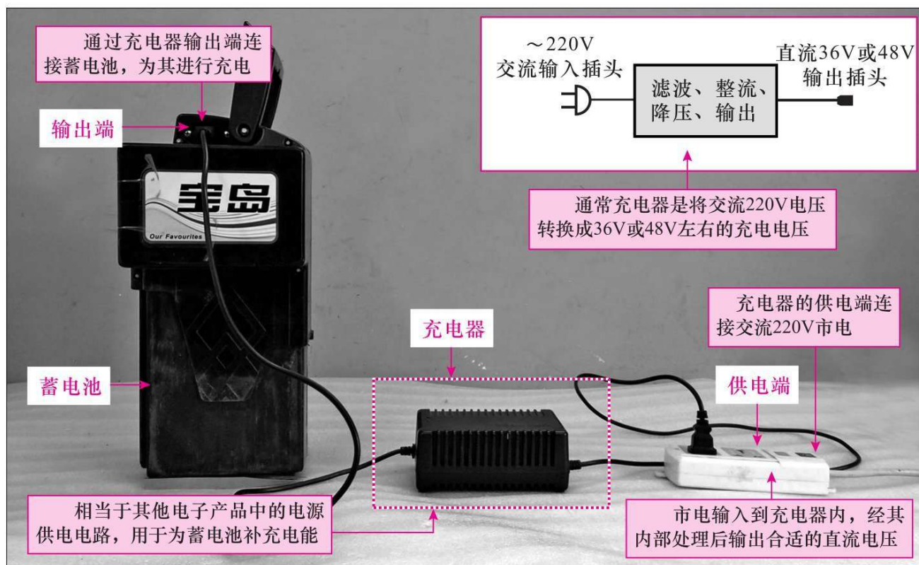
图 1-9 电动自行车中充电器的实物外形
