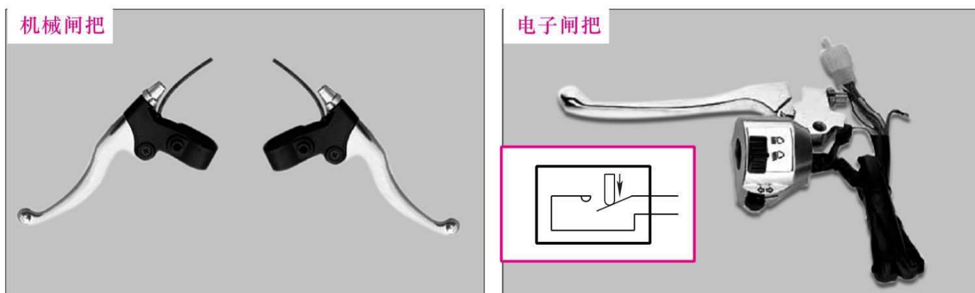
图 1-14 电动自行车中闸把的实物外形
