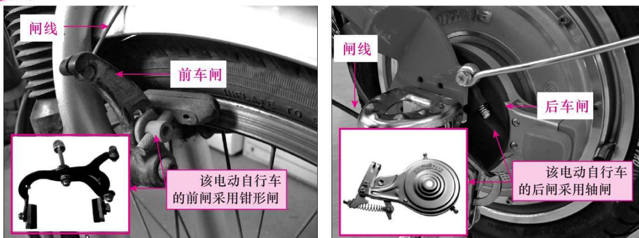
图 1-4 电动自行车的制动部分
