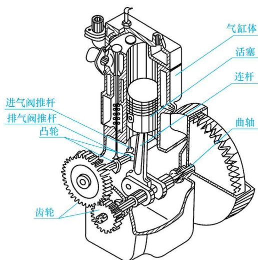
图 1-1 内燃机的发动机局部图
