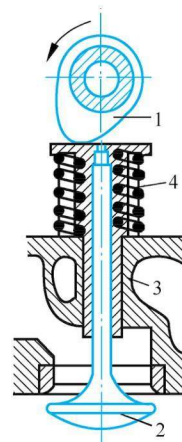
图 1-2 内燃机的配气机构
