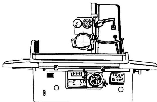
图 1-6 平面磨床
