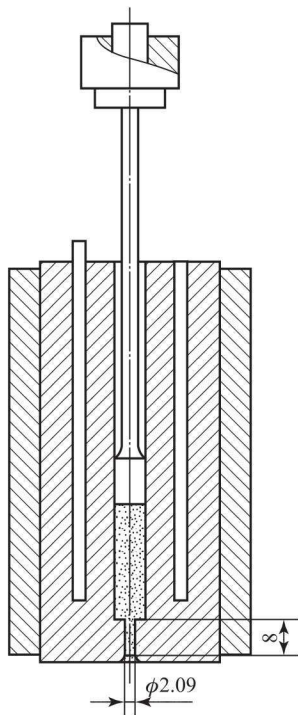
图1-2 熔融指数测定仪结构示意图
