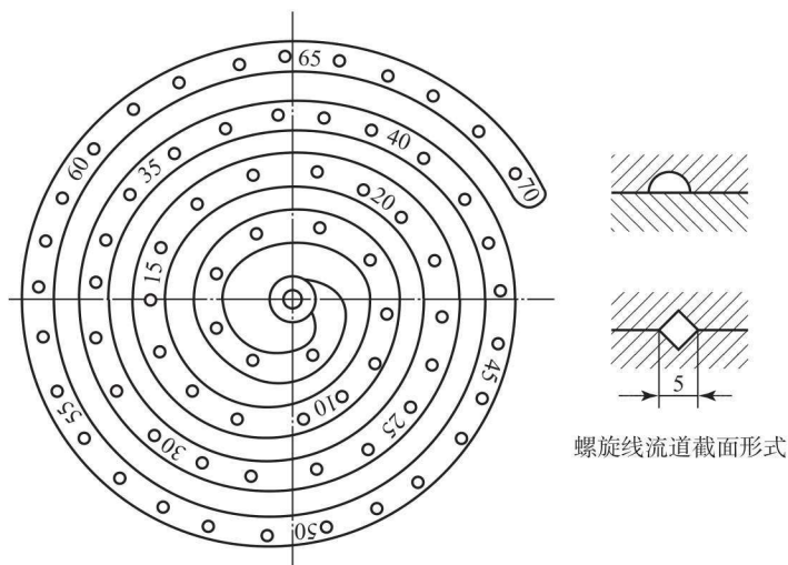
图 1-3 阿基米德螺旋线流动试验模具流道示意图
