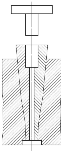
图 1-4 拉西格流动性测定模式示意图
