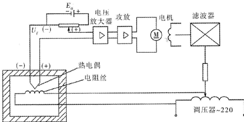
图 1-5 恒温箱的温度自动控制系统
