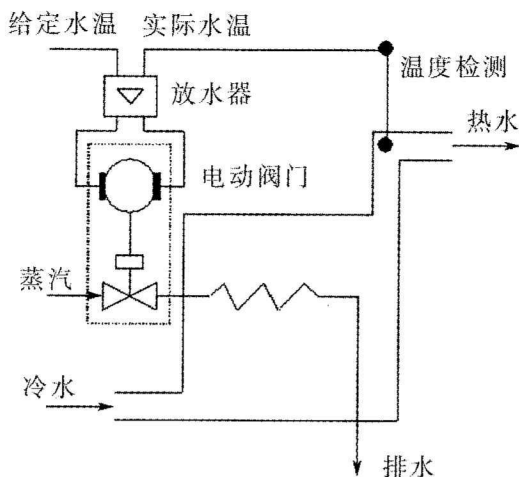
图 1-4 热力控制系统
