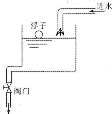
图 1-3 水箱液位自动控制系统
