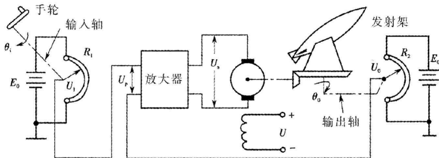
图 1-7 导弹发射架方位角控制系统原理图
