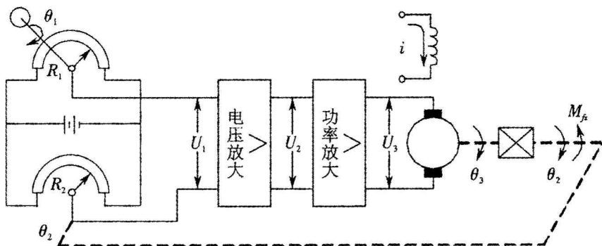
图 1-6 位置随动控制系统
