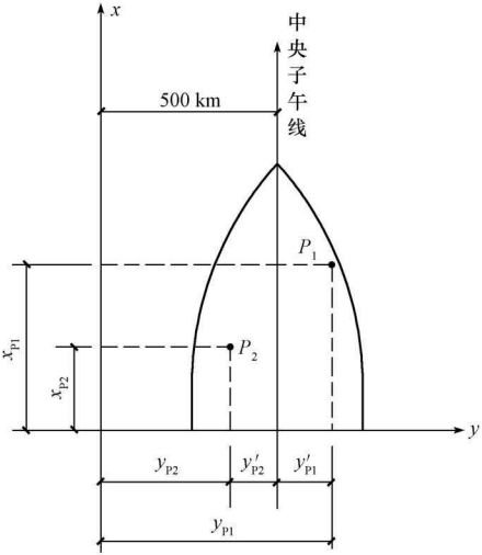
图 1-1-8 高斯平面直角坐标系
