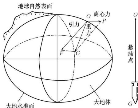
图 1-1-2 假想的静止海洋面
