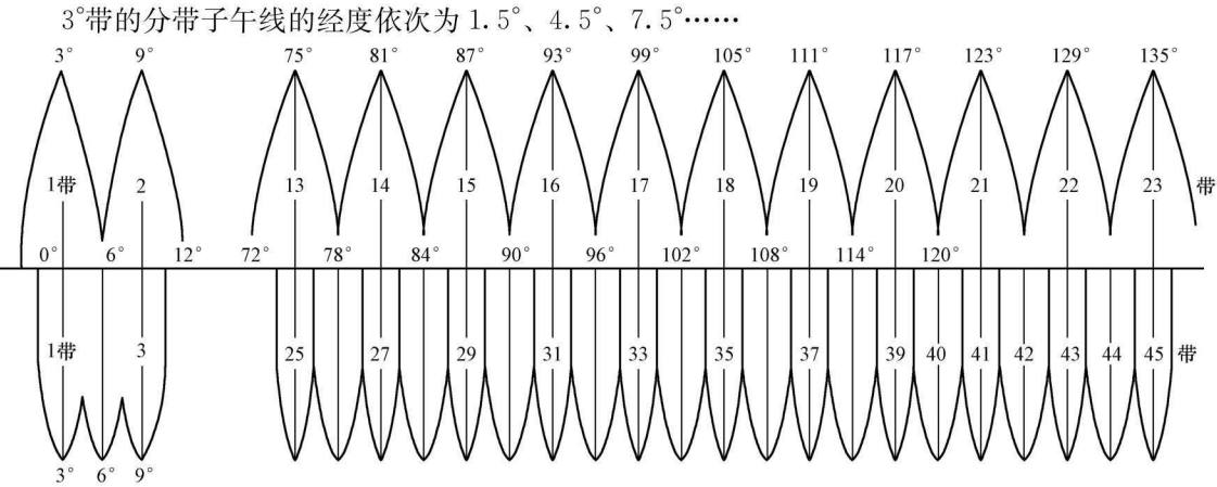
图 1-1-7 6°和 3°投影带的关系
