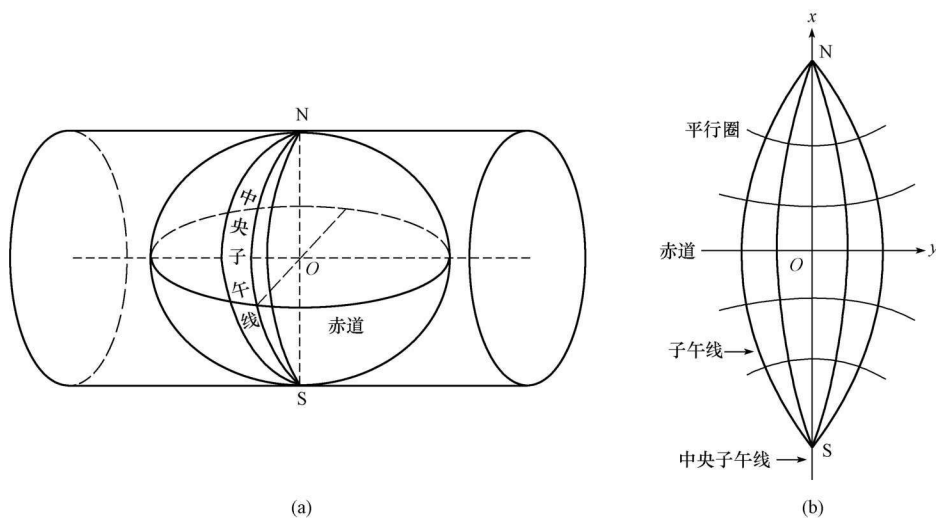
图 1-1-6 横椭圆柱中心投影
