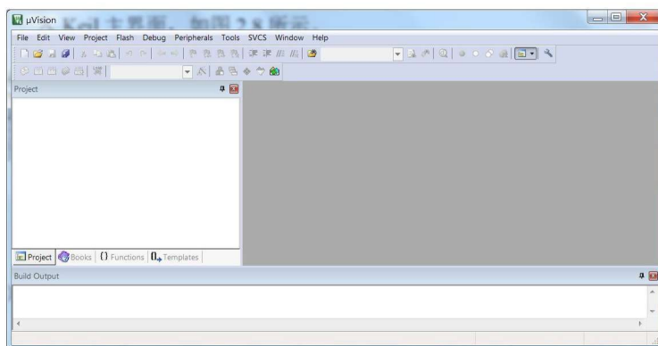
图 2.8 Keil 主界面
