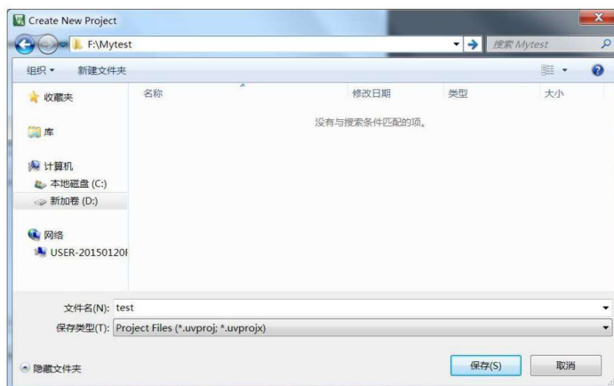
图 2.9 创建工程
