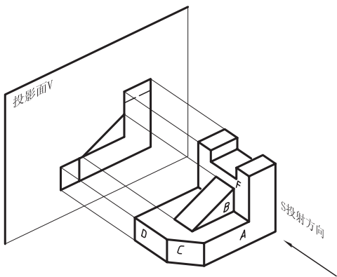
图 2-12 单面投影
