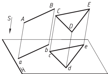
图 2-8 投影面平行线、平行面的投影
