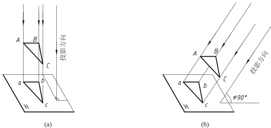
图 2-3 正投影法和斜投影法
