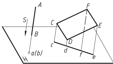
图 2-7 直线、平面的积聚性投影
