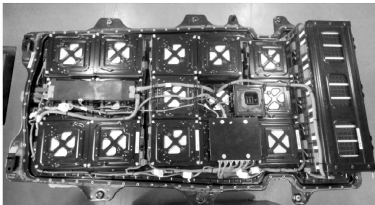
图 1-3 北汽 EV200 纯电动汽车动力电池
