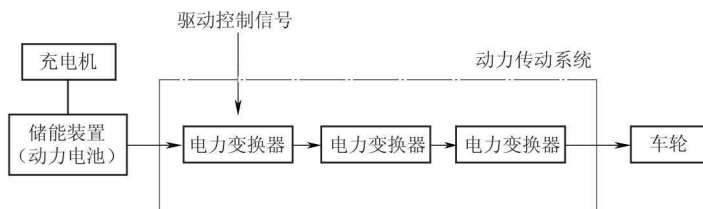
图 1-1 纯电动汽车的系统框图
