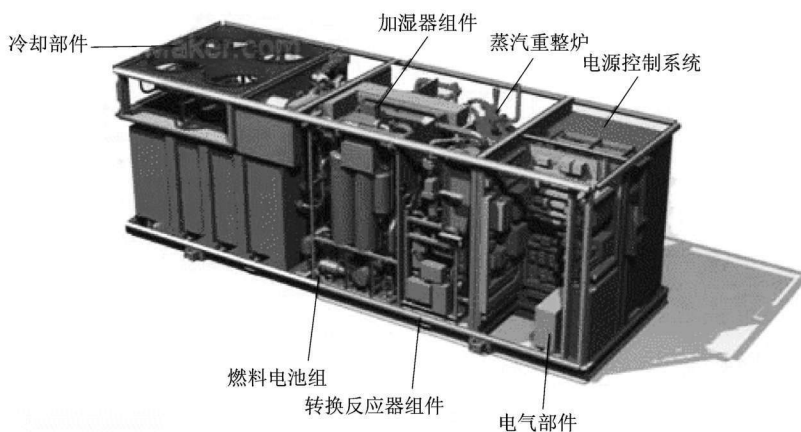
图 1-13 典型的质子交换膜燃料电池
