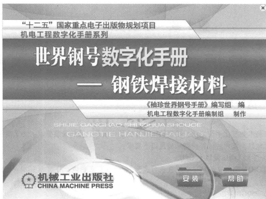
图 1-1 初始界面
