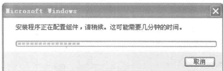
图 1-3 安装进度条
