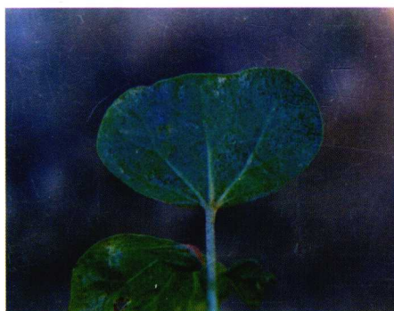
3-13 蓟马危害状
