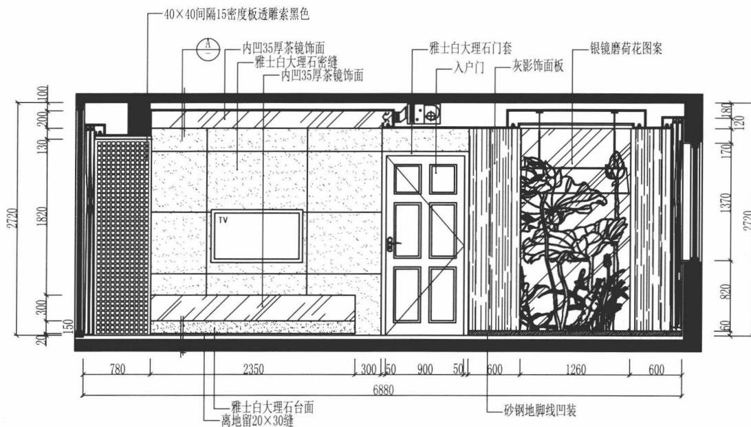
客厅电视墙立面图
