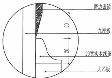
大样图2
