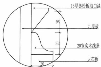
大样图1
