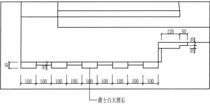
剖面图A
