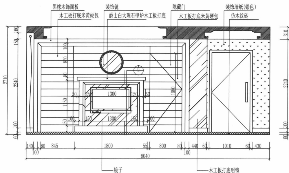
客厅电视墙立面图
