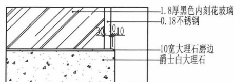
大样图2
