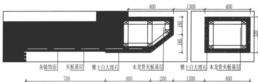
剖面图A
