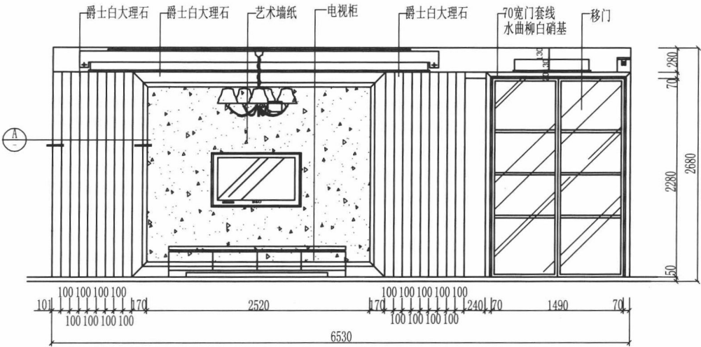
客厅电视墙立面图
