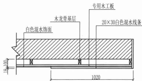
剖面图B
