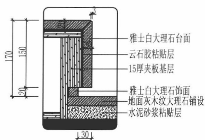
大样图1
