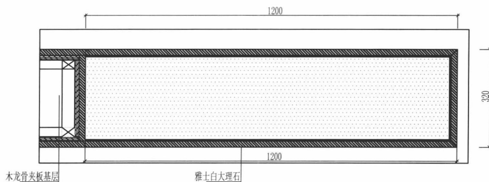
剖面图B
