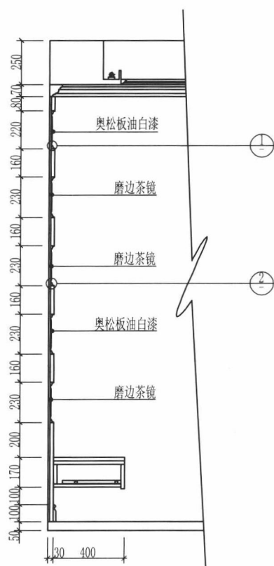
剖面图A
