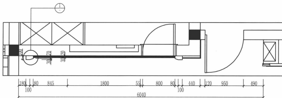
客厅电视墙平面图
