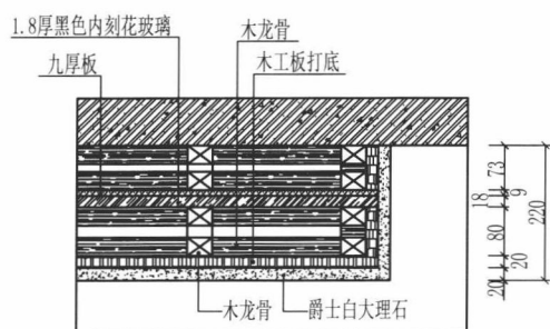
大样图1
