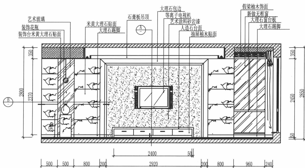
客厅电视墙立面图
