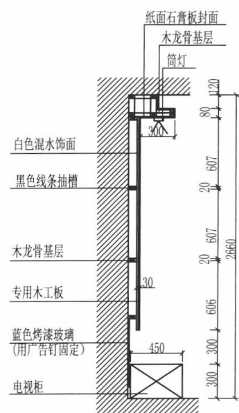
剖面图A
