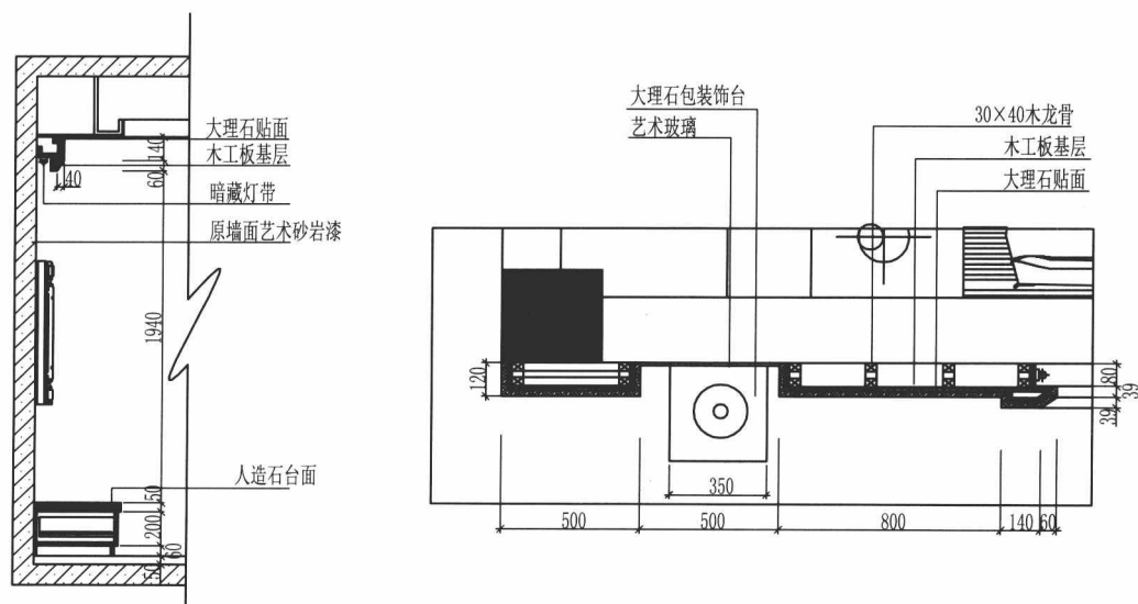
剖面图A
