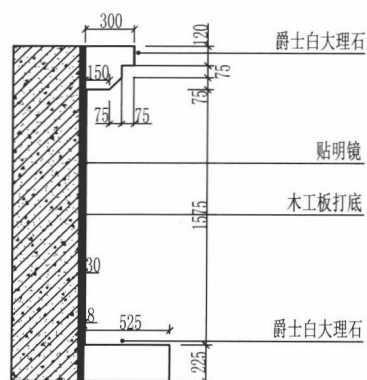
剖面图A
