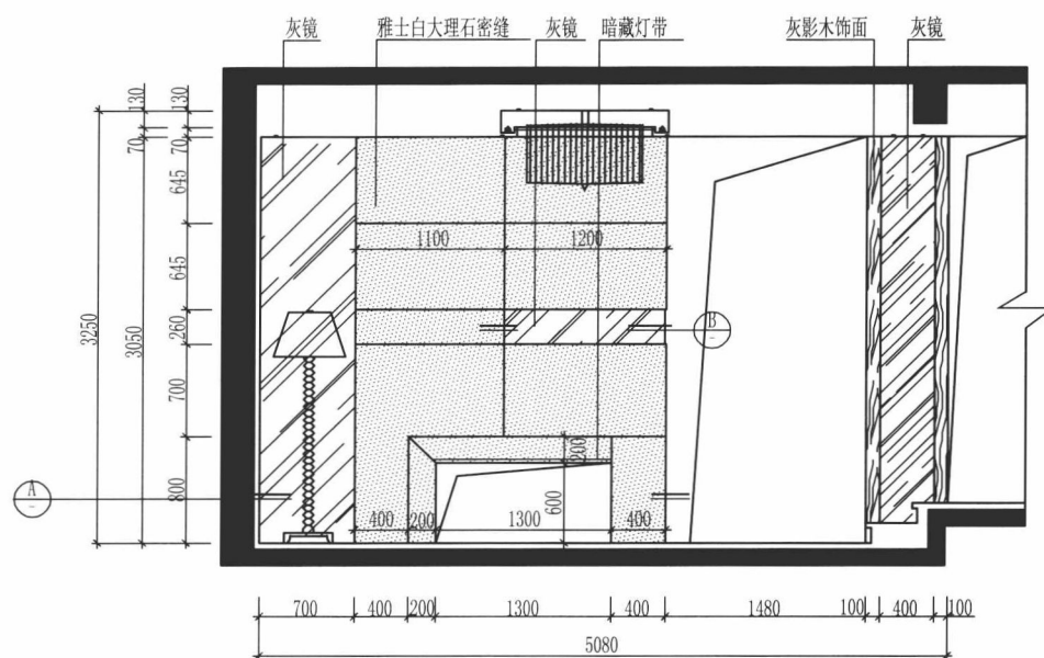
客厅电视墙立面图
