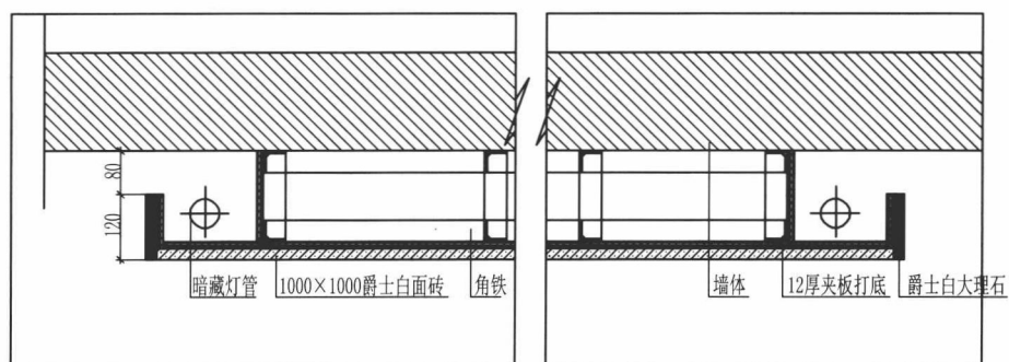
剖面图A
