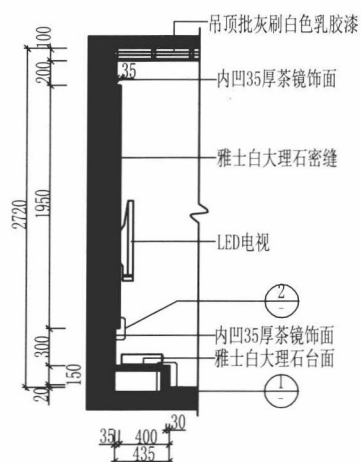
剖面图A
