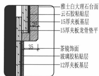
大样图2
