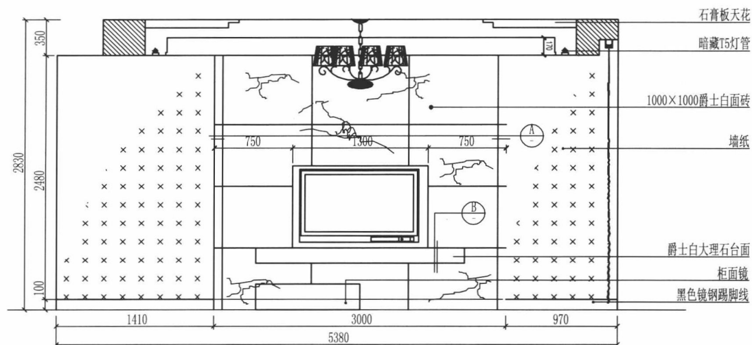
客厅电视墙立面图
