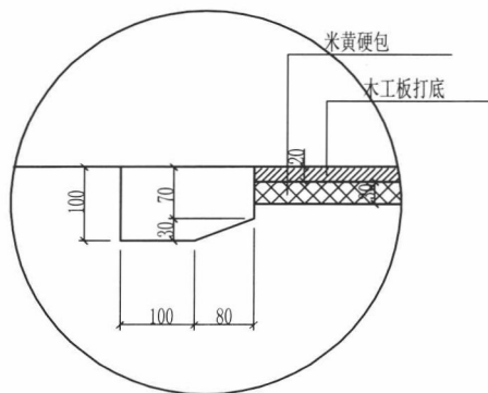
大样图1
