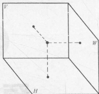
图 1-1 一个点的投影
