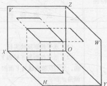
图 1-3 一个几何形的面的投影
