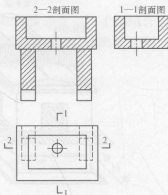
图 1-8 剖面图
