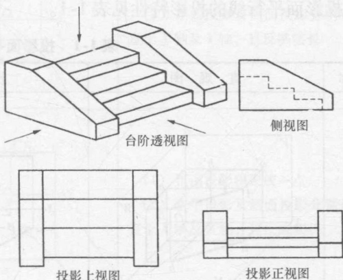
图 1-4 台阶外形的投影
