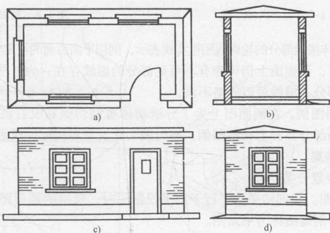
图 1-6 房屋的剖切视图
