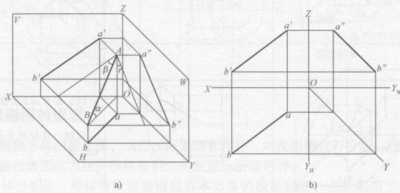
图 1-5 一般位置直线的投影 a) 直观图 b) 投影图
