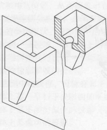
图 1-7 剖面图的形成
