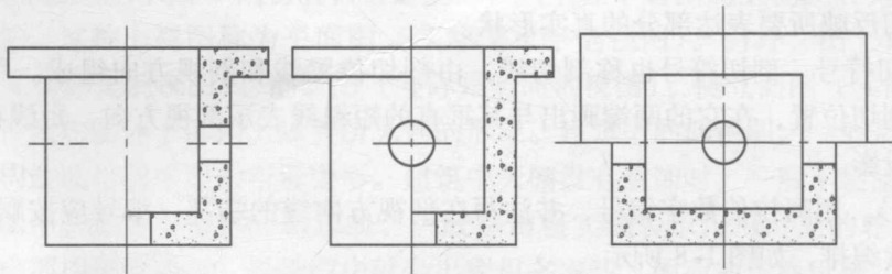
图 1-9 半剖面图
