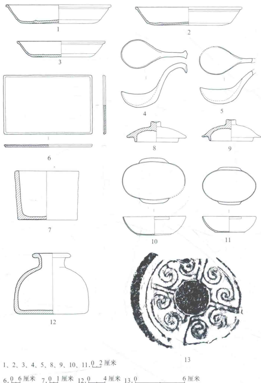
图六 IM4070 出土陶器
