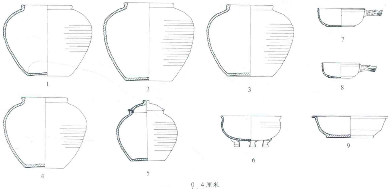
图五 IM4070 出土陶器
