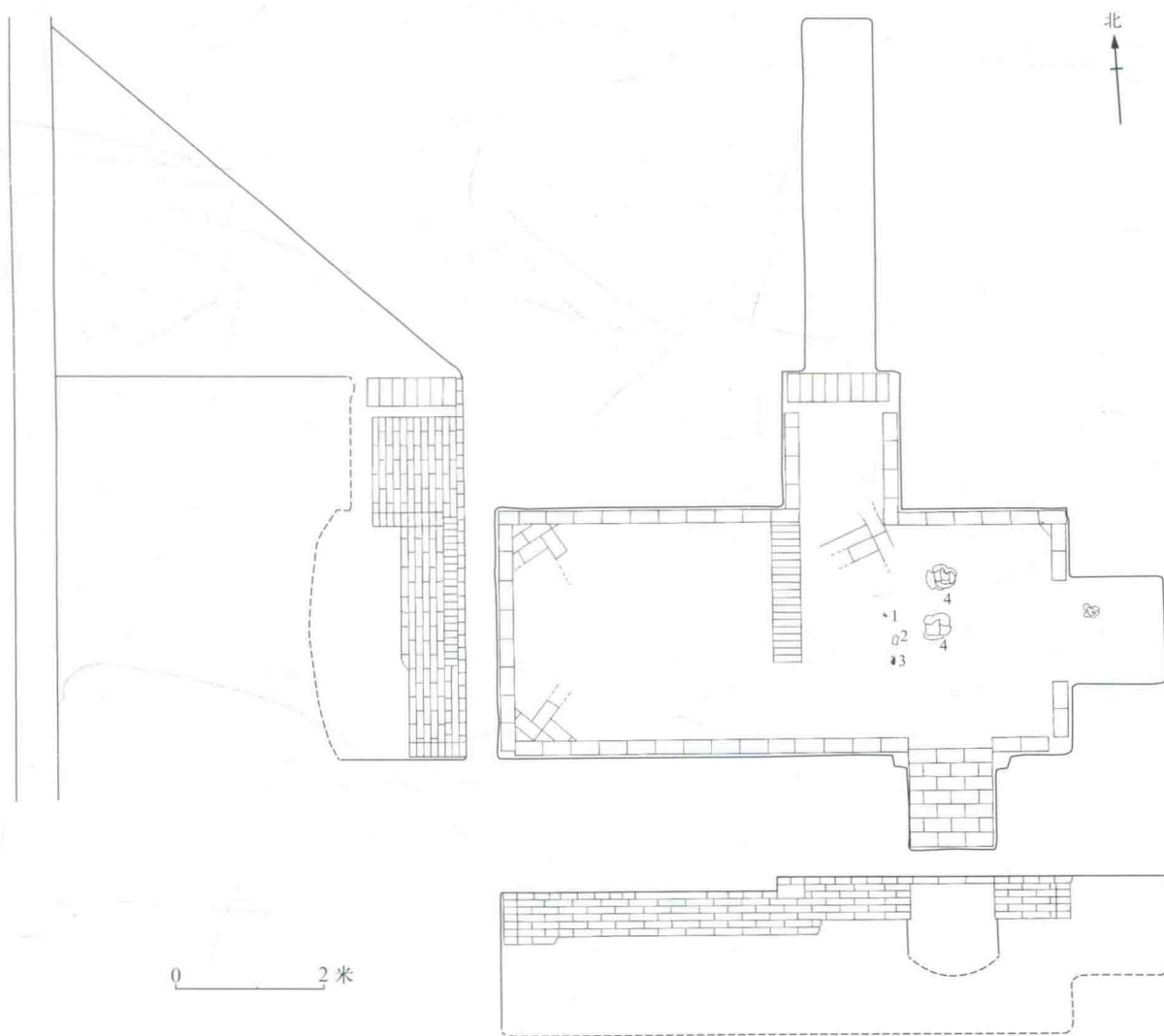
图一〇 IM4169 平、剖面图
