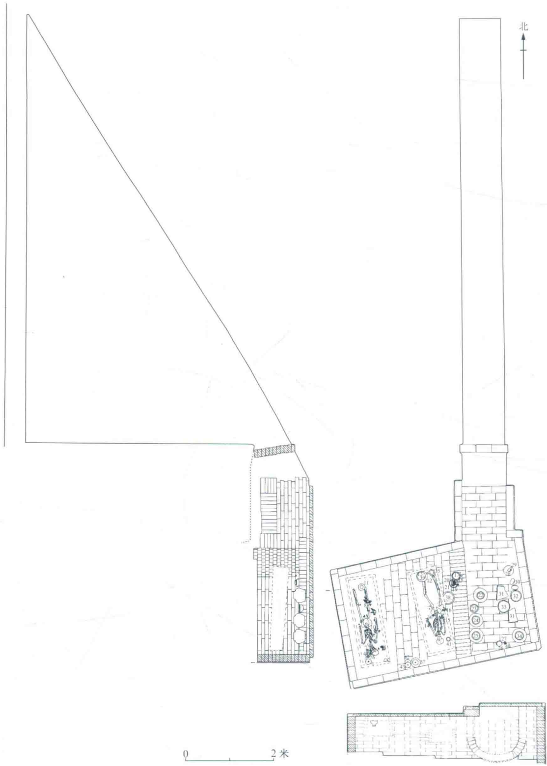
图二 IM4070 平、剖面图
