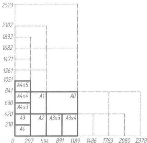
图 1-1 图纸基本幅面及加长幅面尺寸
