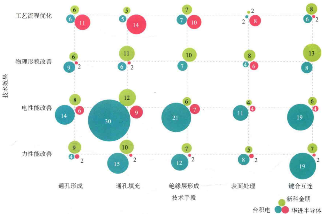
图6-2-10 华进半导体、台积电、新科金朋硅通孔制造工艺技术功效图
