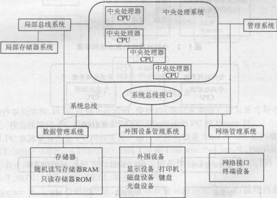
图 1-1 巨型和大中型计算机的基本结构示意图
