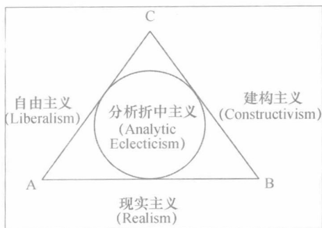
图2 综合性三角解释模型 ①
