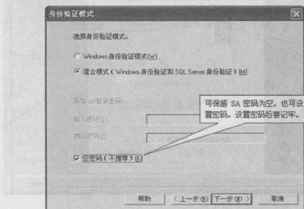
图 1-6 身份验证模式
