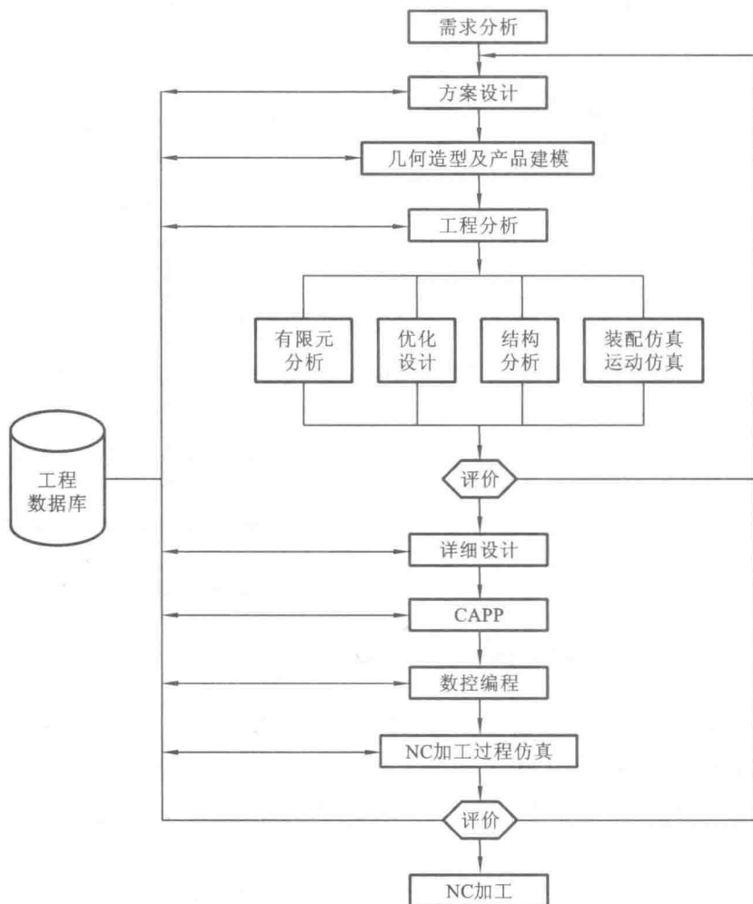
图 1.1 机械产品设计和制造的流程图
