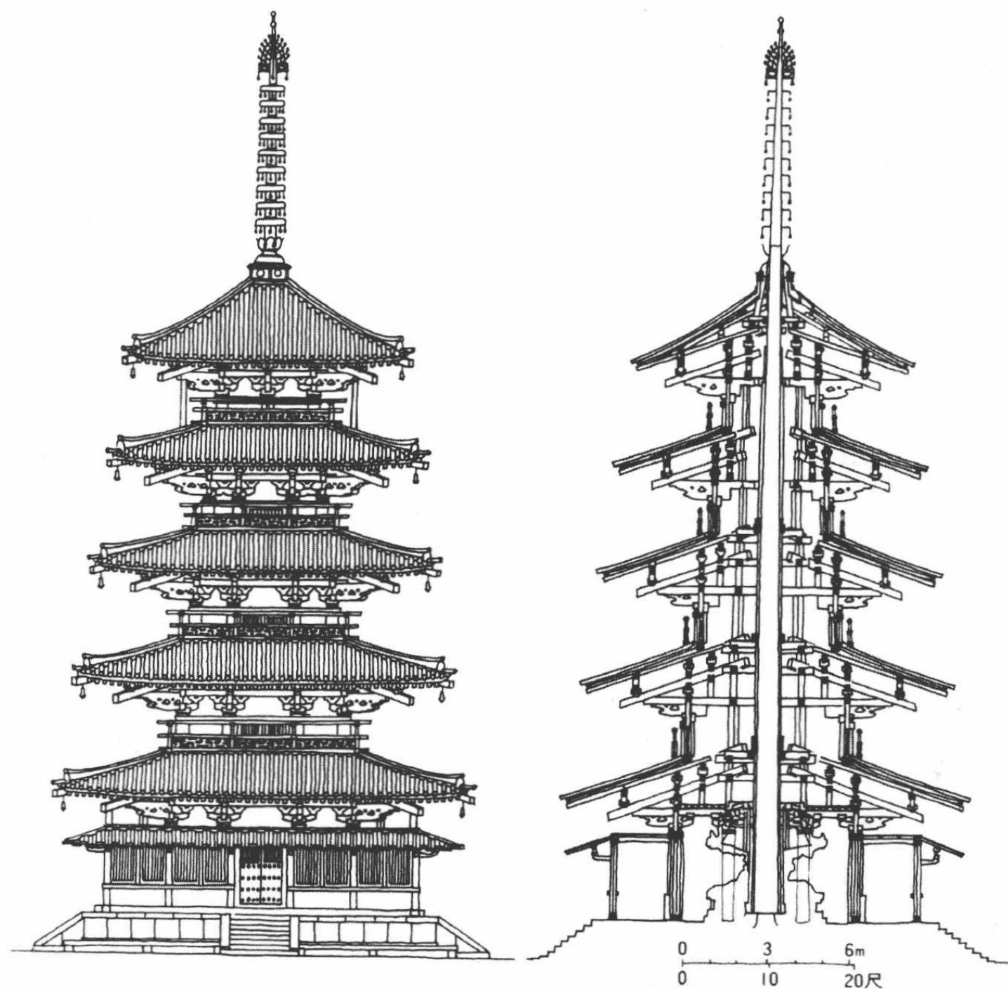
法隆寺五重塔 立面图、剖面图
