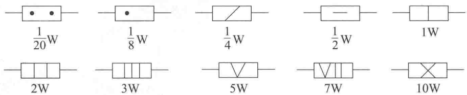
图 2-2 额定功率的符号表示法
