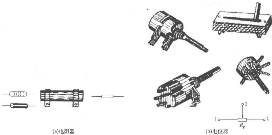
图 2-1 常用电阻器外形及符号
