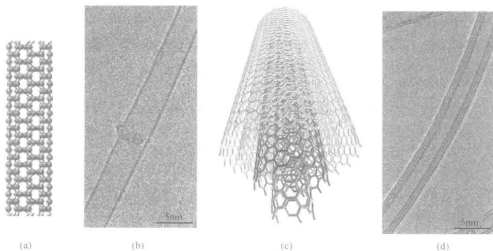
图1-2 单壁碳纳米管的示意图(a)和其透射电镜照片(b);多壁碳纳米管的示意图(c)和其透射电镜照片(d) [7]
