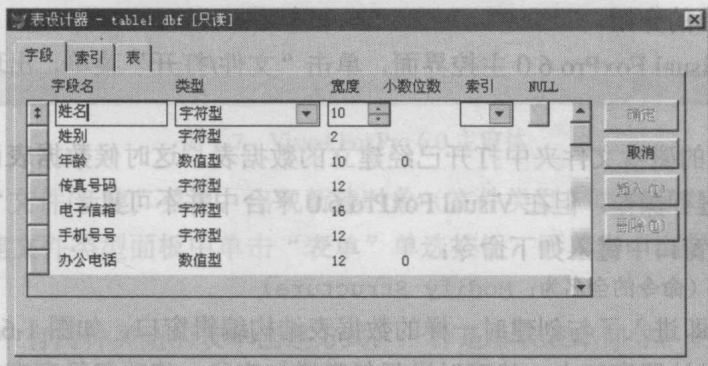
图 1-6 表结构的实际创建
