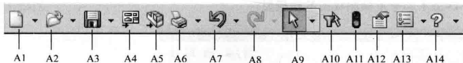
图 1.3.2 “常用”工具栏
