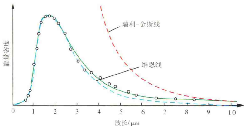
图 2-2 黑体辐射实验值(小圆圈)与两个公式的理论值(虚线)的图示, 维恩公式只适用于短波部分, 瑞利-金斯公式只适用于长波部分
