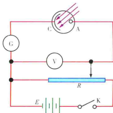
图 2-3 光电效应实验装置示意图
