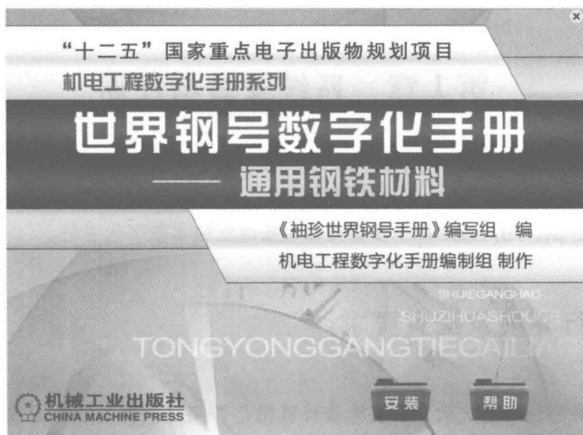
图 1-1 初始界面
