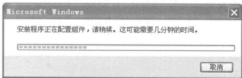
图 1-3 安装进度条
