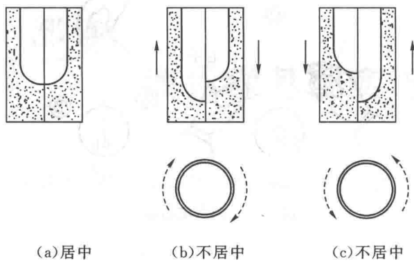
图 1-4 精确整平
