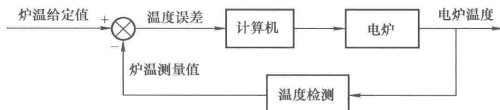
图 1-12 电炉温度控制系统框图
