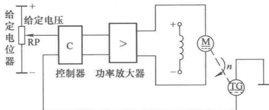
图 1-7 电动机转速自动闭环控制系统
