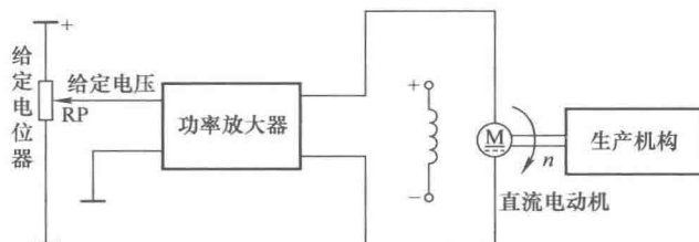
图 1-4 直流电动机转速开环控制系统
