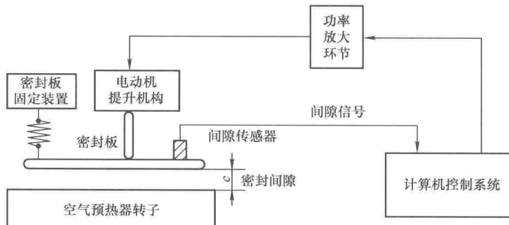
图 1-13 电站锅炉空气预热器密封间隙控制系统
