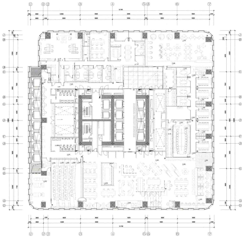
一层平面图
