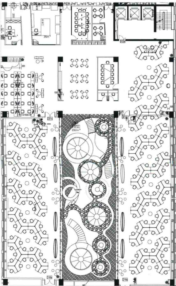
一层平面图
