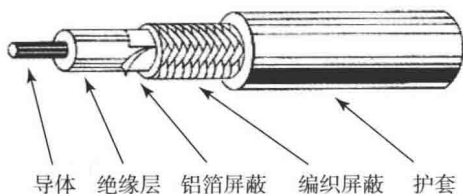
图 1.2.1 同轴电缆的结构
