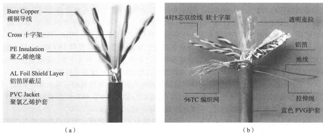
图 1.2.4 4 对双绞线电缆结构
