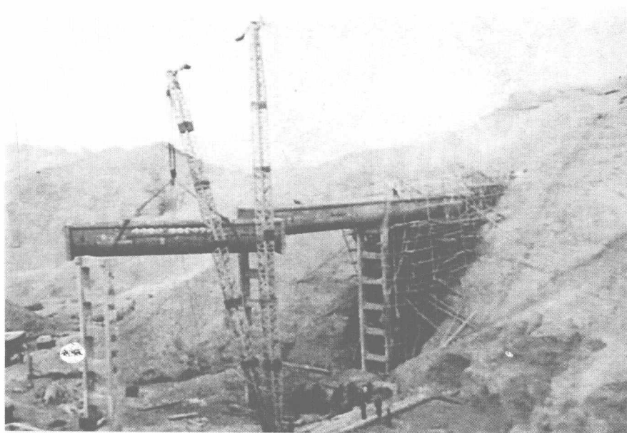
土法吊装
