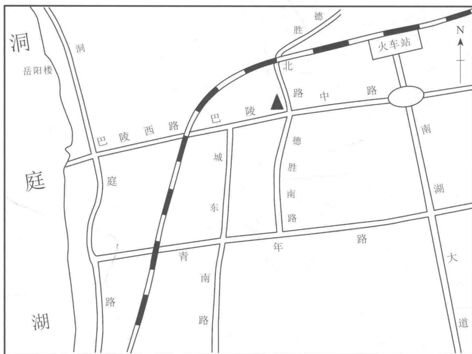
图 1-1-1 桃花山古墓群位置示意图
