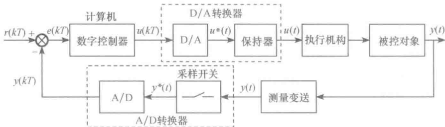
图 1.2 计算机控制系统典型结构
