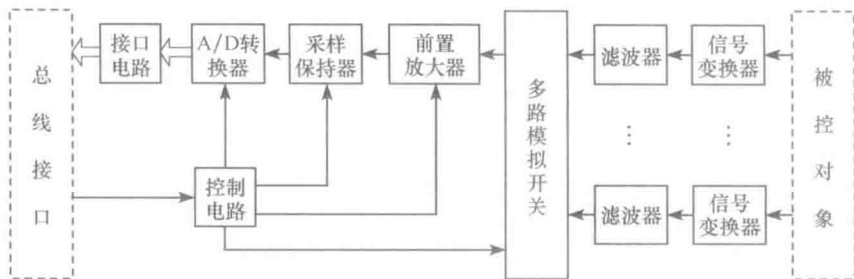
图 1.4 模拟量输入通道组成与结构图
