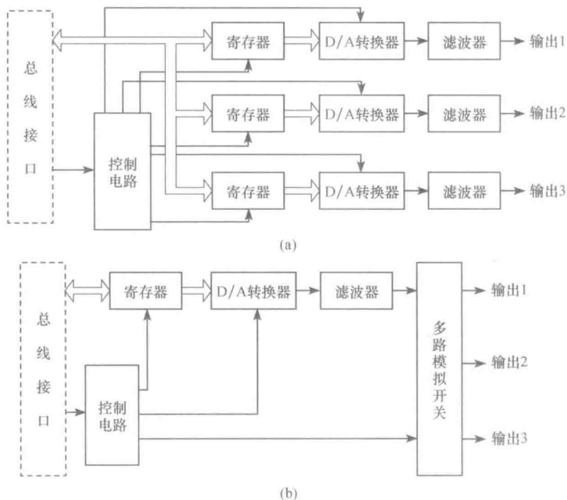
图 1.5 模拟量输出通道组成与结构图
