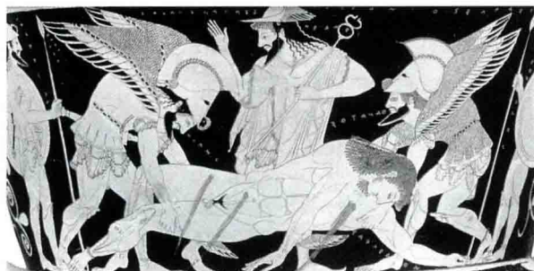
图1-10 希腊瓶画
