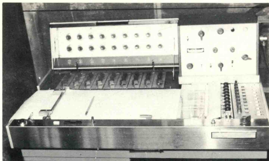
MD—95 D型八频道检查仪
