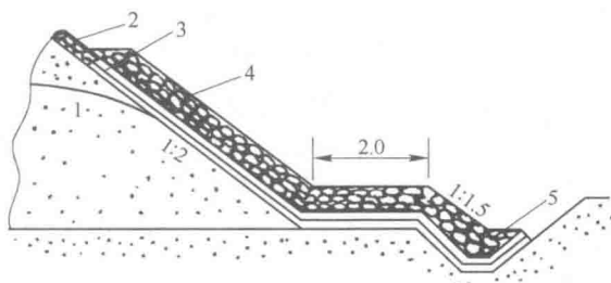
图 2F311012-3 贴坡排水 (单位: m)
