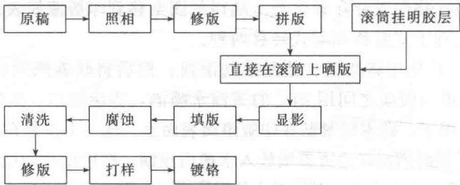
图 1-4 照相网点凹版制版工艺流程
