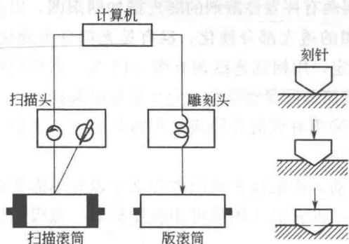
图 1-7 电子雕刻机工作原理示意图
