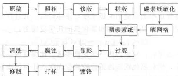
图 1-3 照相凹版间接制版工艺流程
