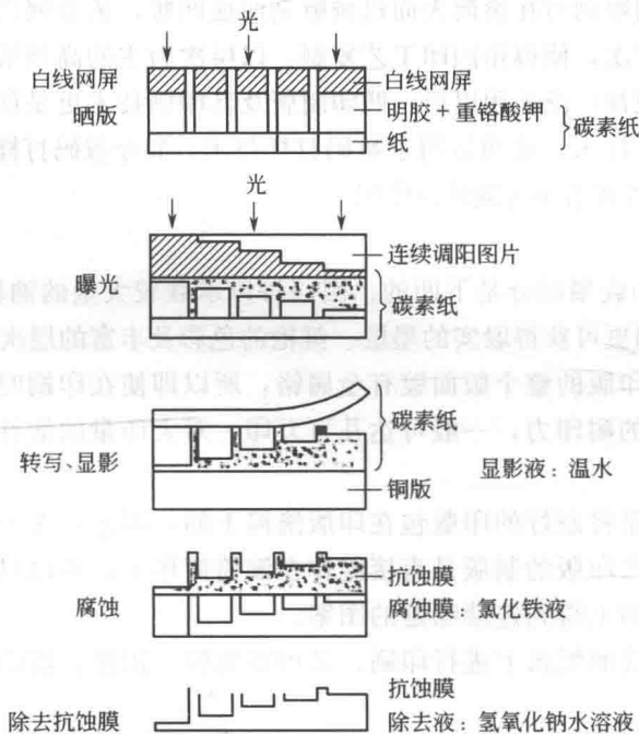
图 1-1 间接制版工艺过程
