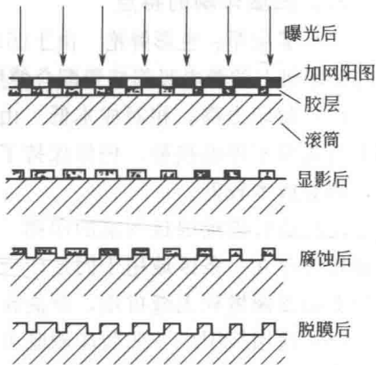
图 1-2 直接制版工艺过程
