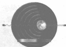
多普勒红移
