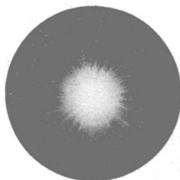
宇宙大爆炸
