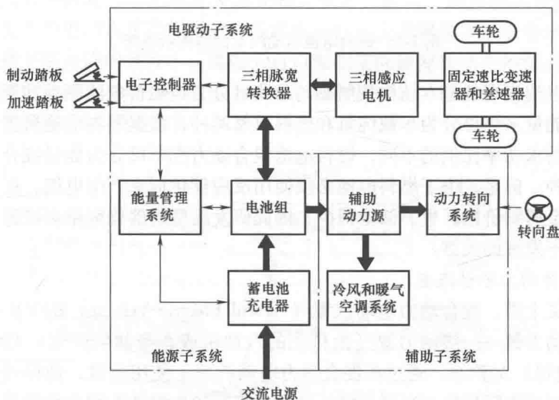
图 1-1 典型的纯电动汽车结构示意图
